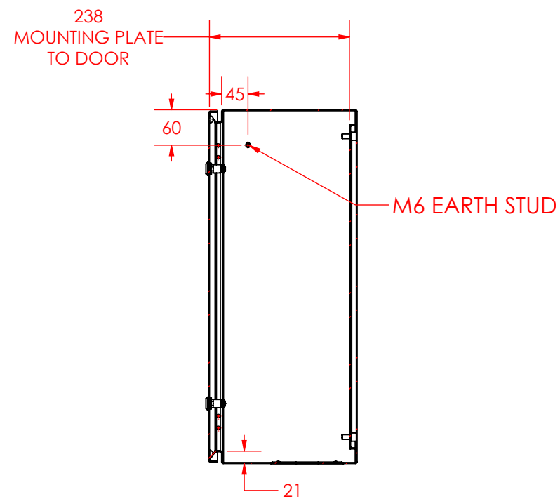
SECTION A-A SCALE 1 : 9
