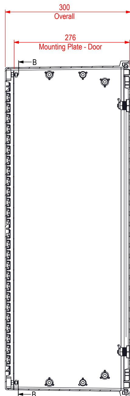
SECTION A-A
