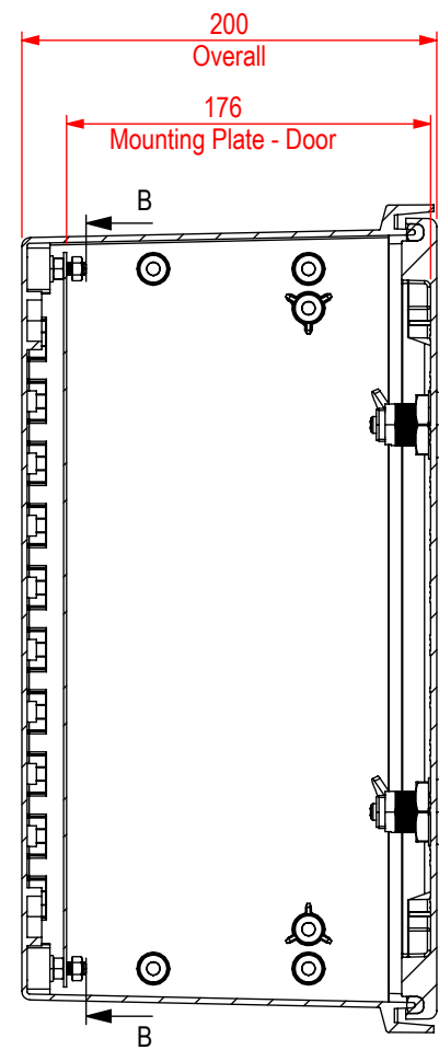
SECTION A-A
